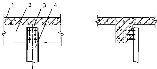
图 9 支架与梁固定示意
