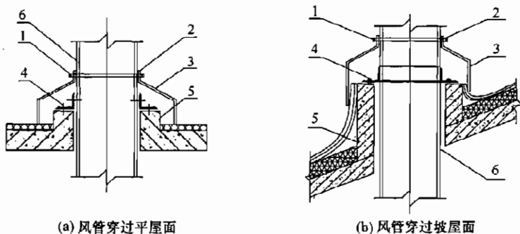
图 8.1.9 风管穿屋面防雨渗漏装置示意
