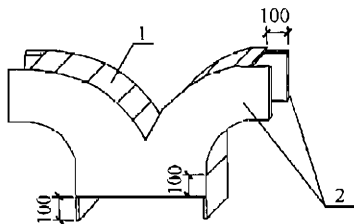
图 5.4.2-4 蝴蝶三通放样下料示意
