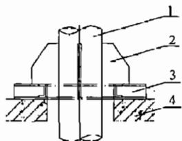
图 15 双侧挡板式固定支架示意
