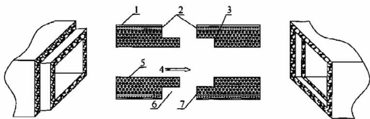
图 8.3.6-1 承插阶梯粘接接口示意
