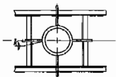
图 16 穿楼板管道
