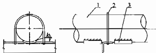
图 14 带弧形挡板管卡式固定支架示意
