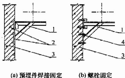
图 11 斜支撑型支架示意
