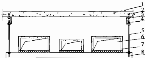
图 22 水平布置多风管共用吊架示意
