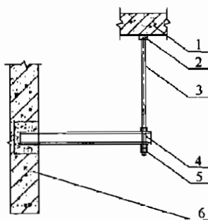
图 13 支架一端固定 端悬吊安装示意
