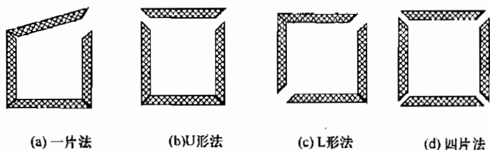
图 5.2.2-1 矩形风管 45°角组合方式示意
