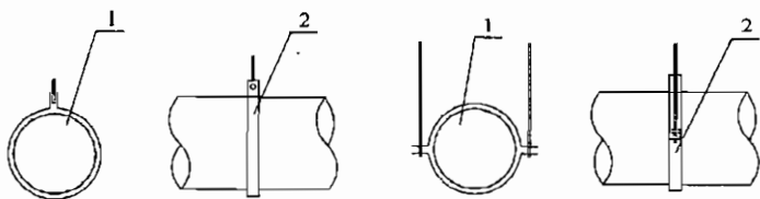
图 7.2.5-3 柔性风管吊环安装
