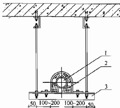
图 7.2.5-2 水管横担预留长度示意
