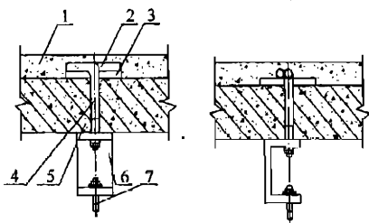
图 8 穿楼板螺栓固定示意
