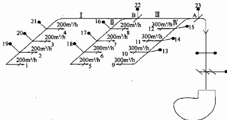
图 35 送风系统图
