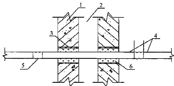
图 11.1.4-2 水管过结构变形缝墙体安装示意
