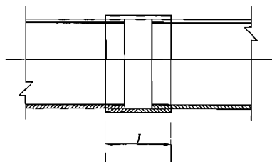
图 5.5.7-2 软接头示意
