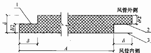
图 5.3.2-3 风管承插阶梯粘接示意
