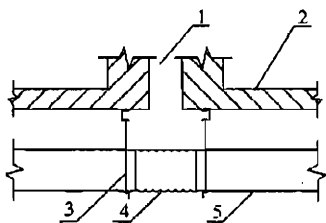
图 8.4.3-1 风管过变形缝空间的安装示意
